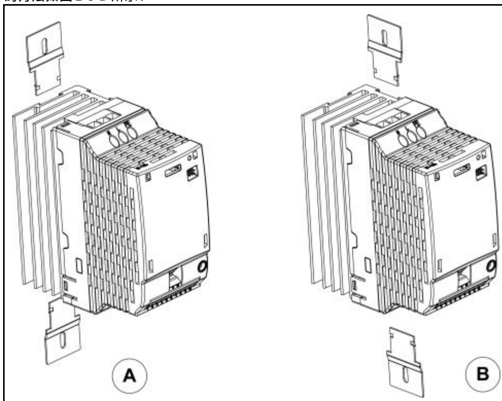
图 2-6 安装支架
