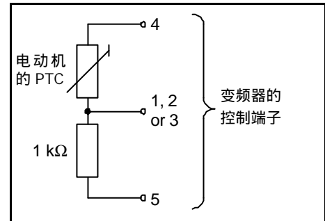
图 3-8 电动机过载保护的 PTC 接线
