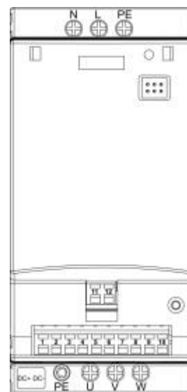
图 2-8 MICROMASTER 410 变频器的接线端子
