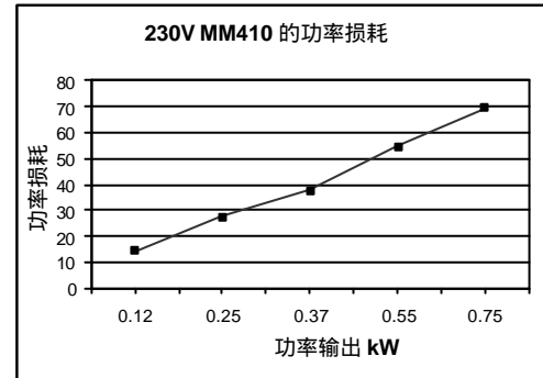
图 2-2 功率损耗，230 V
