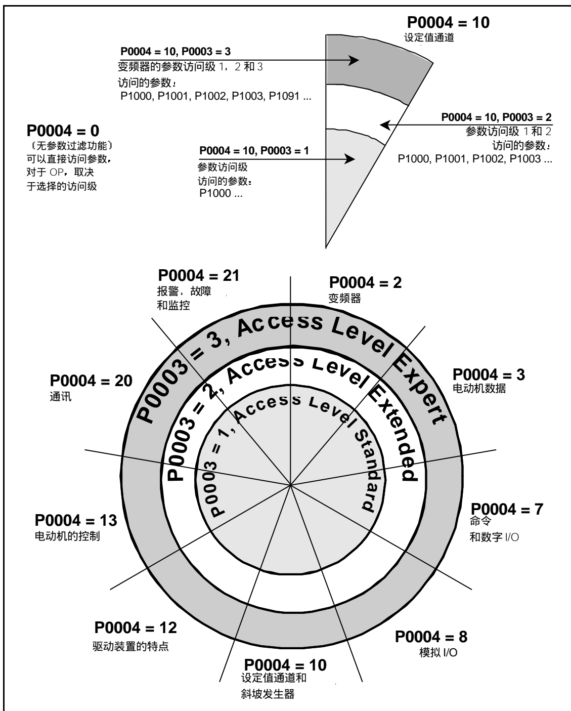
图 5-1 参数概览
